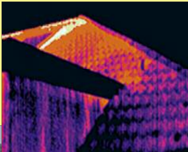
Die Thermografie zeigt mit roter Färbung Wärmeverluste an Gebäudeaußenseiten. Schwachstellen befinden sich häufig im Bereich von Dachfenstern, Gauben oder der gesamten Dachhaut.
